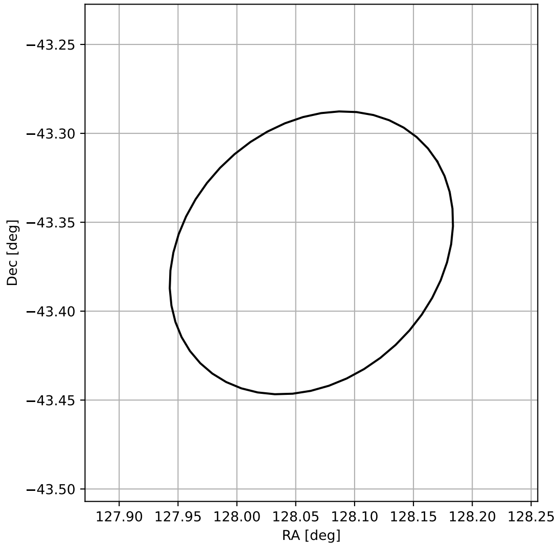
4FGL J0832.2-4322
