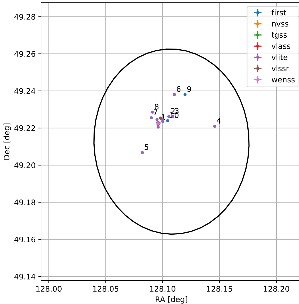
4FGL J0832.4+4912
