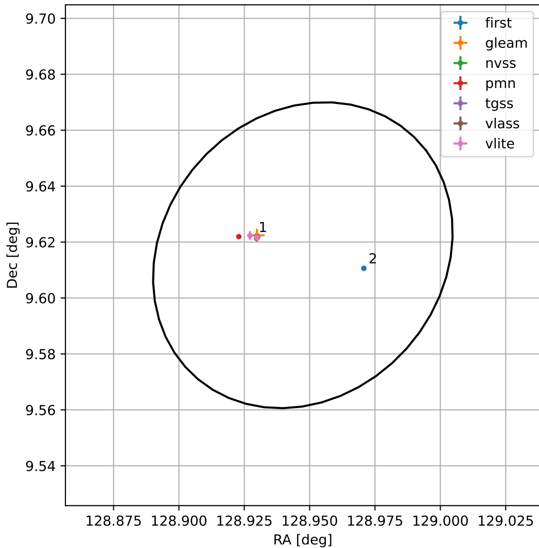
4FGL J0835.7+0936
