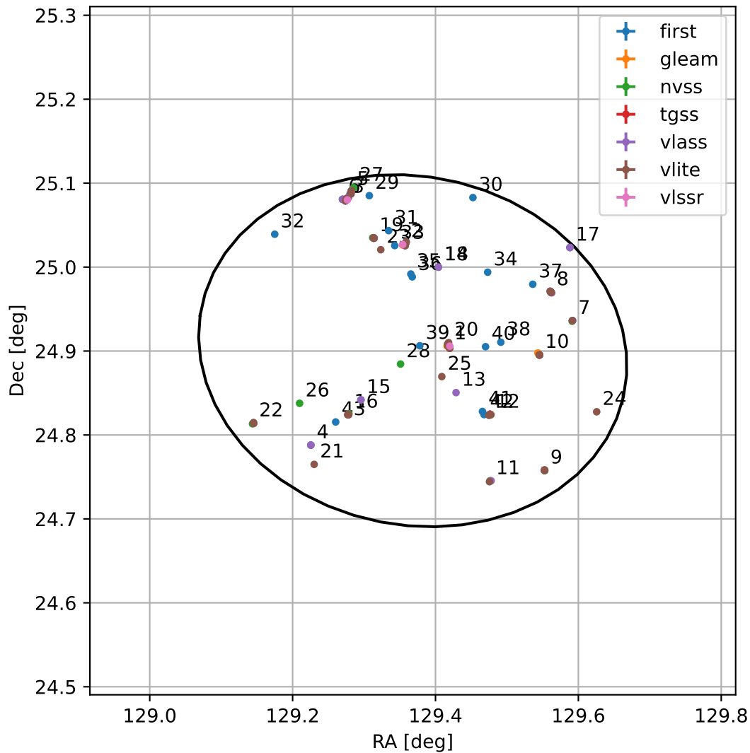
4FGL J0837.4+2454
