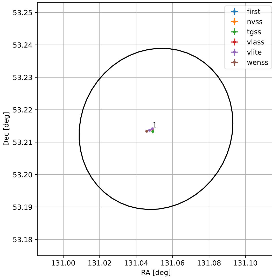
4FGL J0844.2+5312
