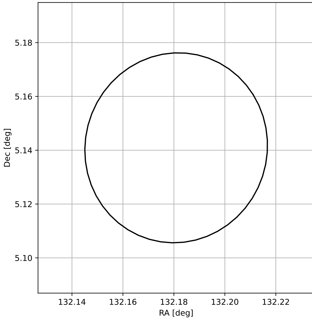
4FGL J0848.7+0508
