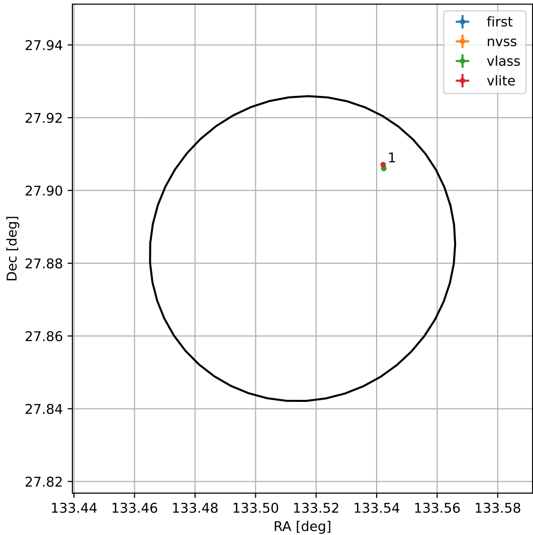
4FGL J0854.0+2753
