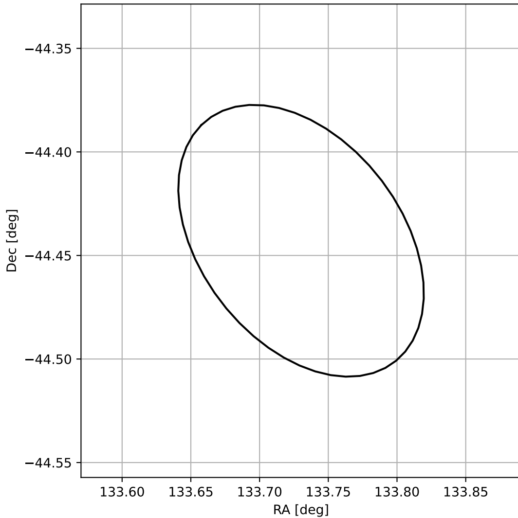
4FGL J0854.9-4426
