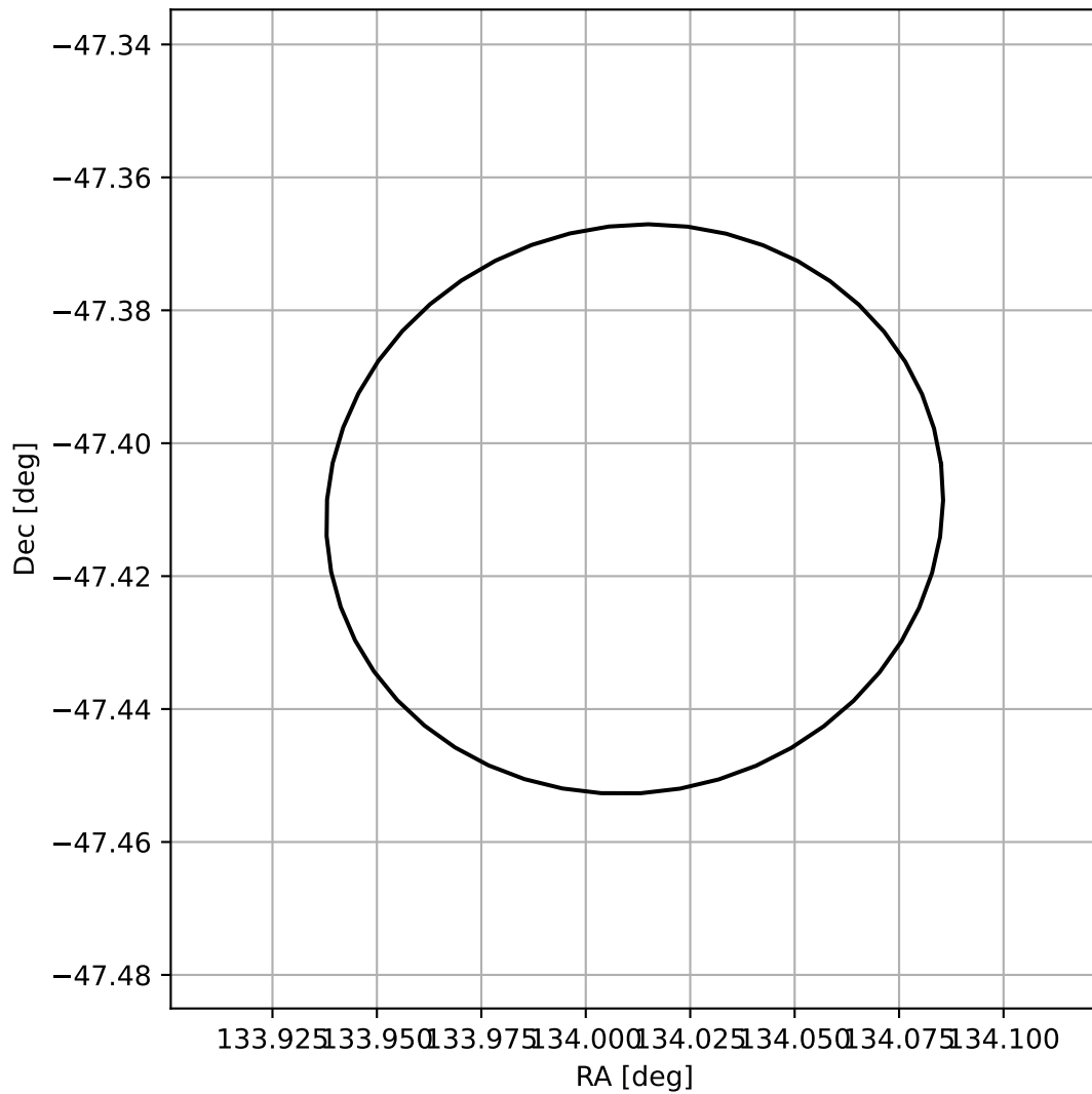
4FGL J0856.0-4724
