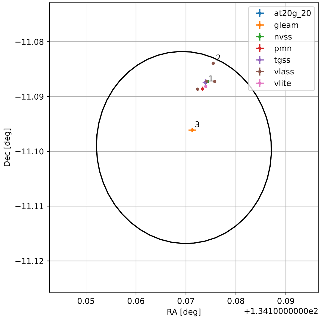
4FGL J0856.6-1105
