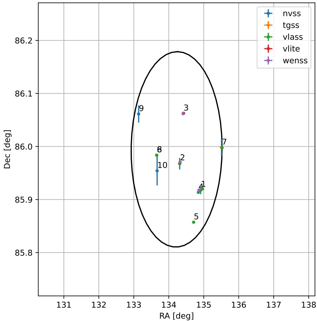
4FGL J0856.8+8559
