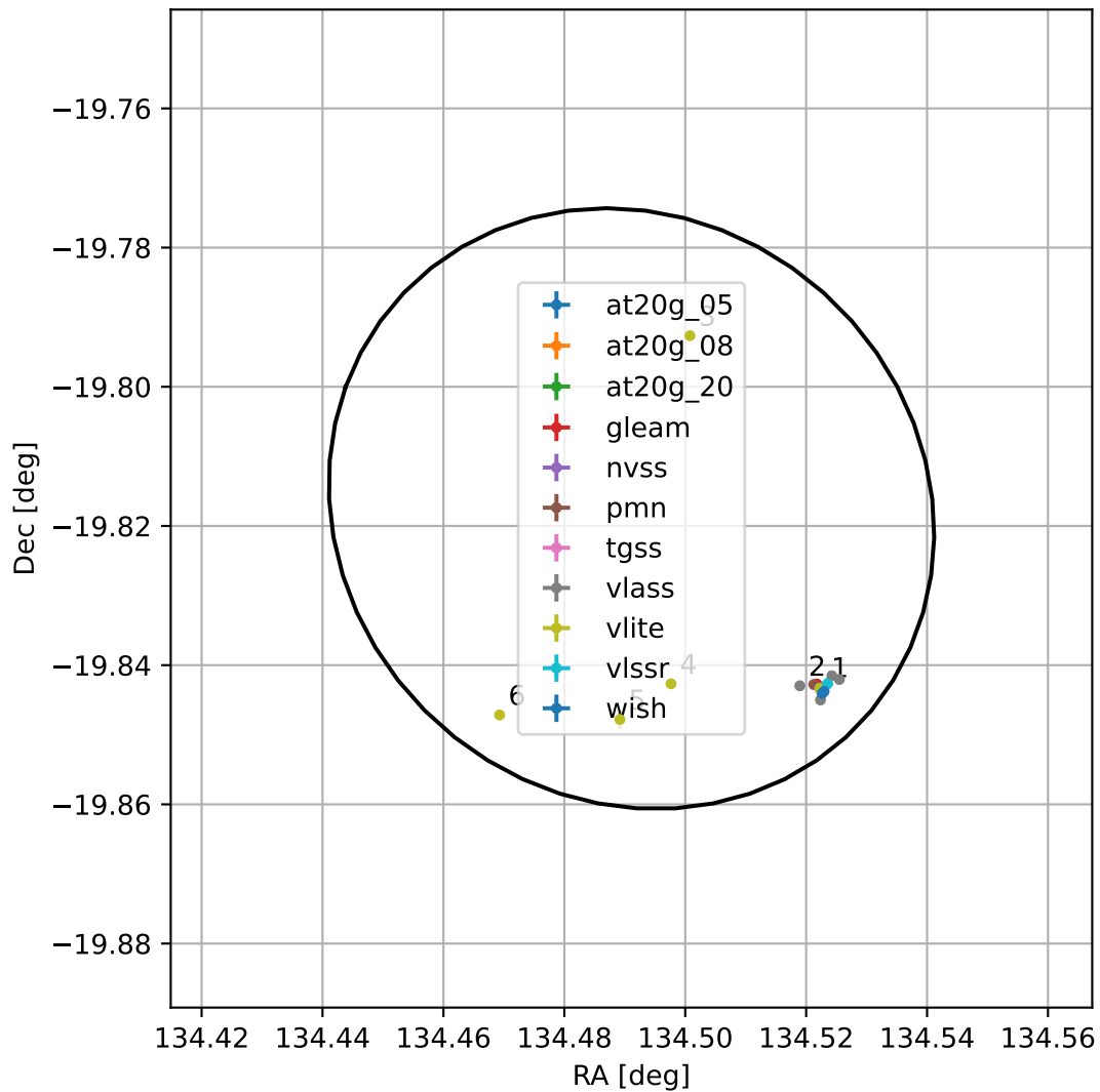
4FGL J0857.9-1949
