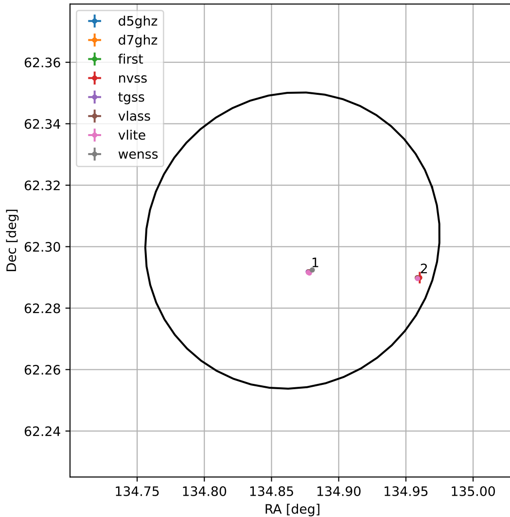
4FGL J0859.4+6218
