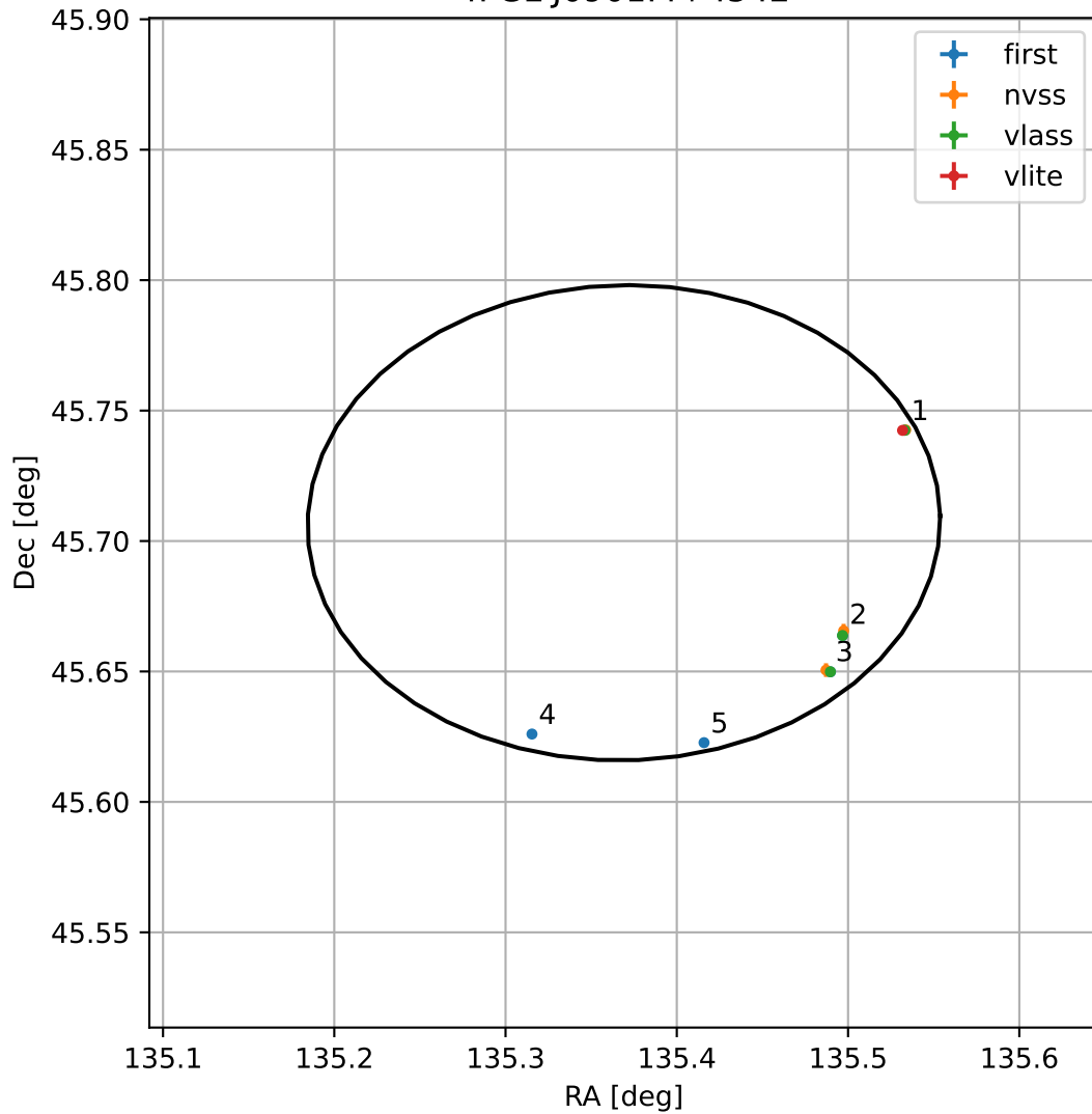
4FGL J0901.4+4542
