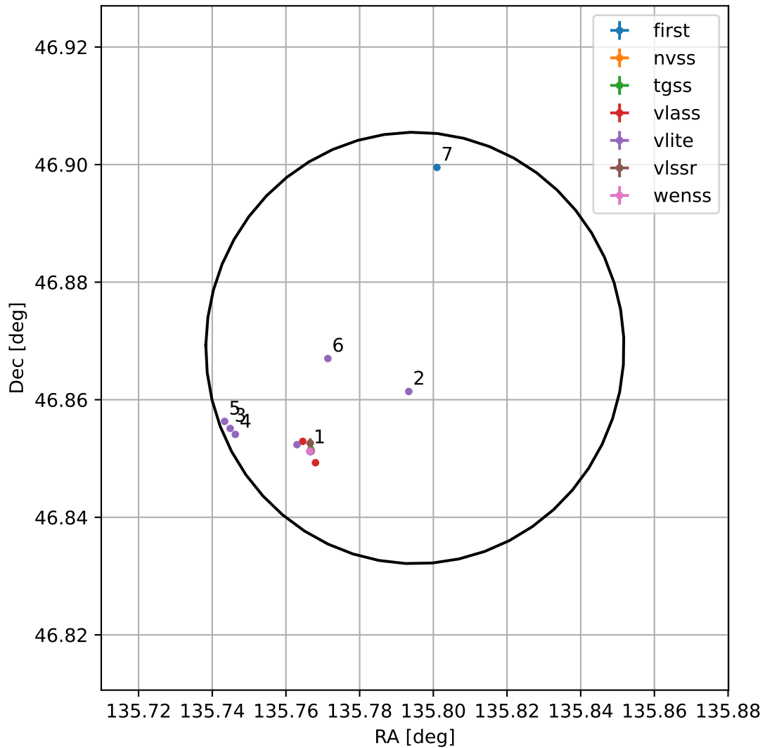
4FGL J0903.1+4652
