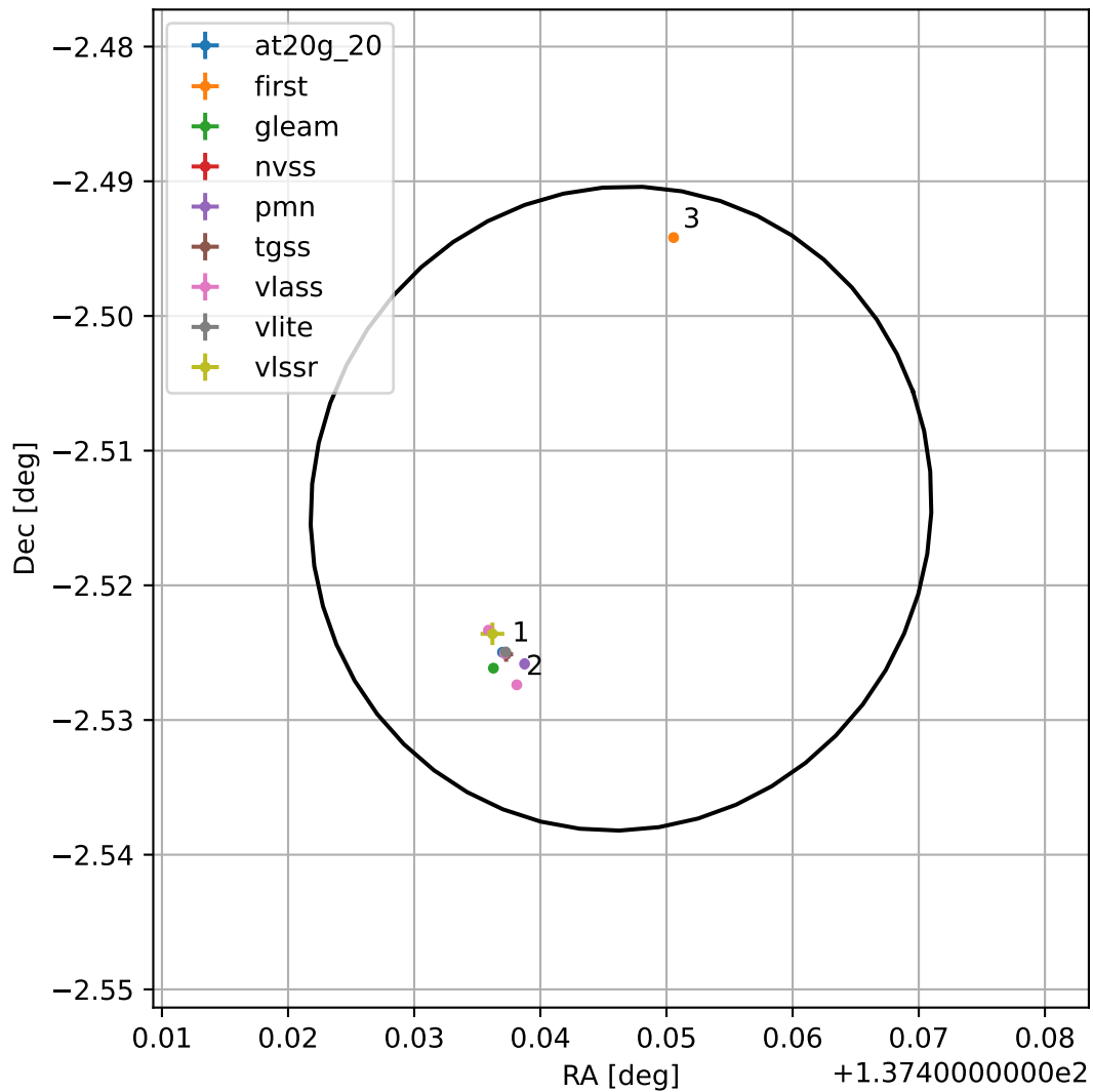
4FGL J0909.7-0230
