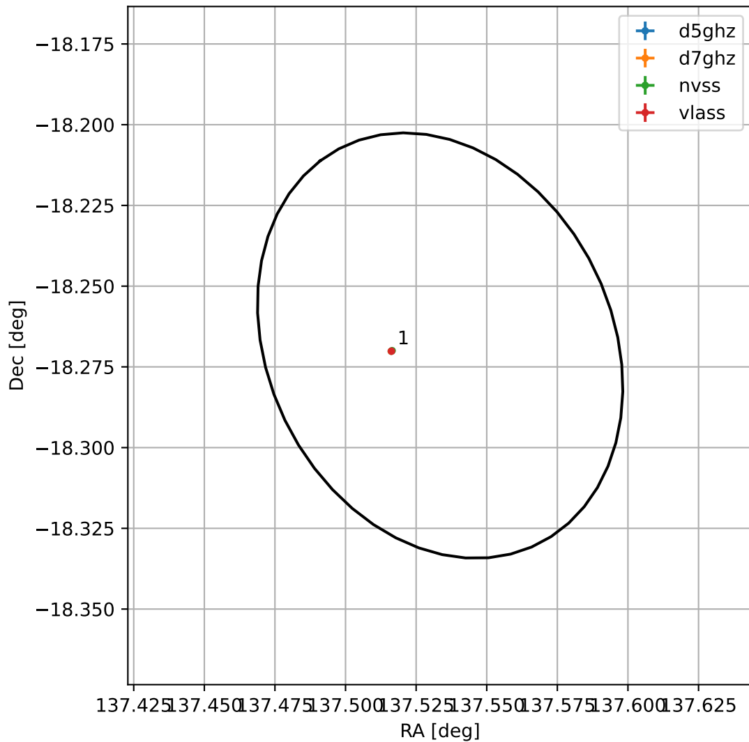
4FGL J0910.1-1816
