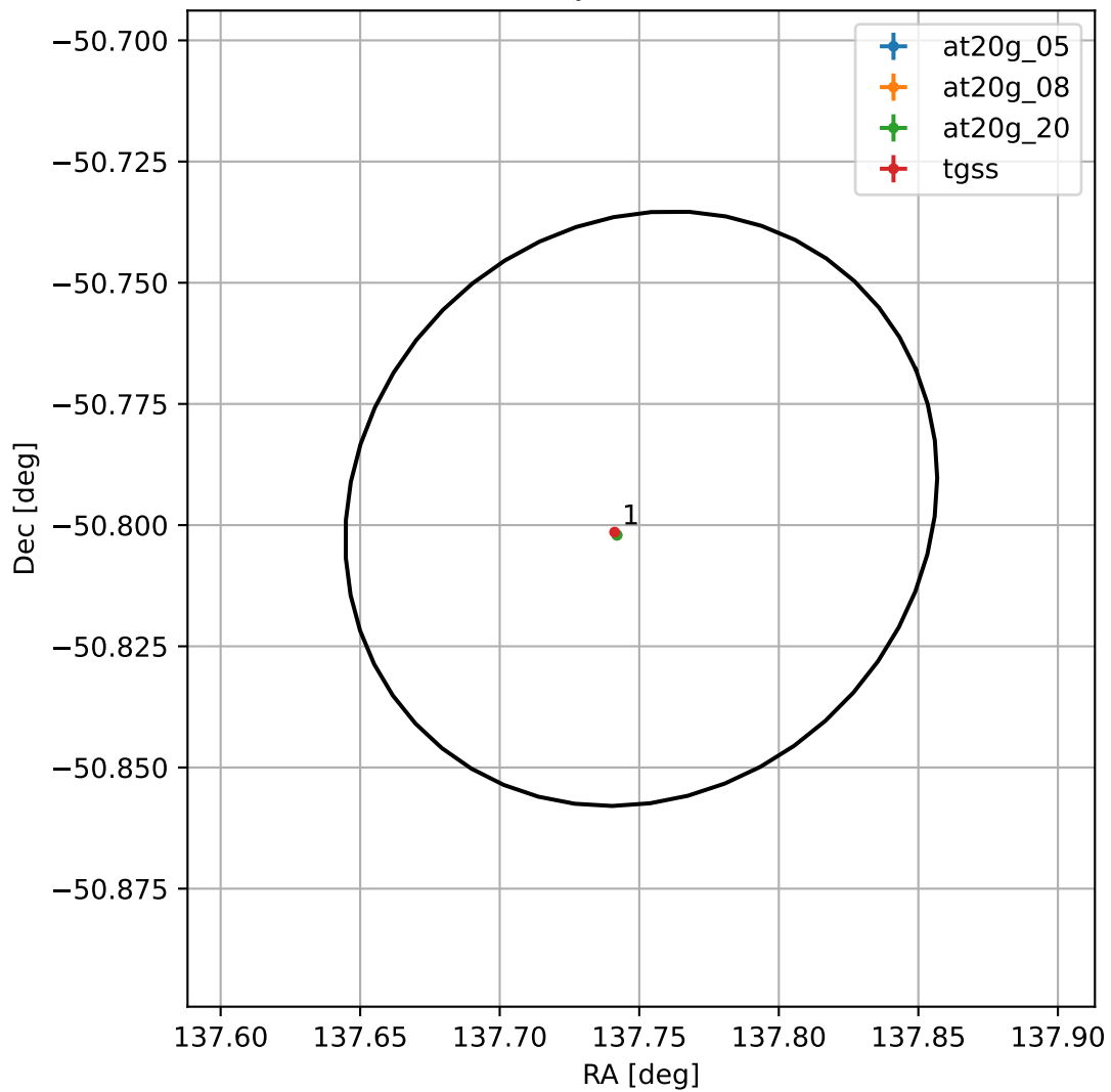
4FGL J0911.0-5047
