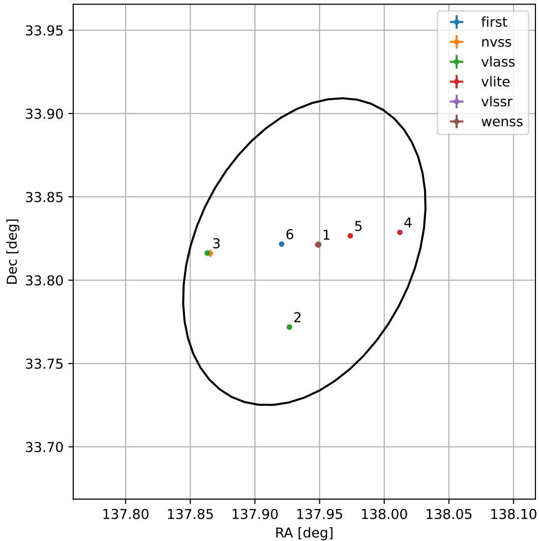
4FGL J0911.7+3349
