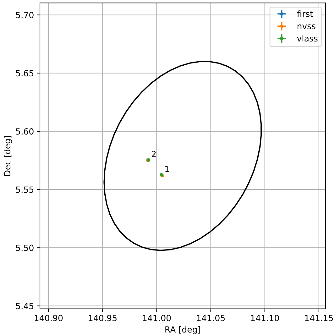
4FGL J0924.0+0534
