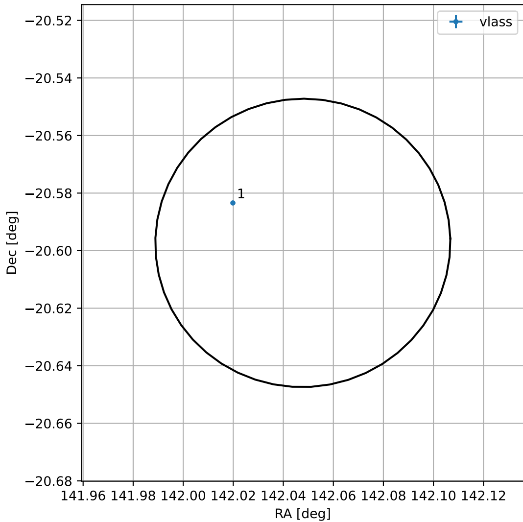
4FGL J0928.1-2035
