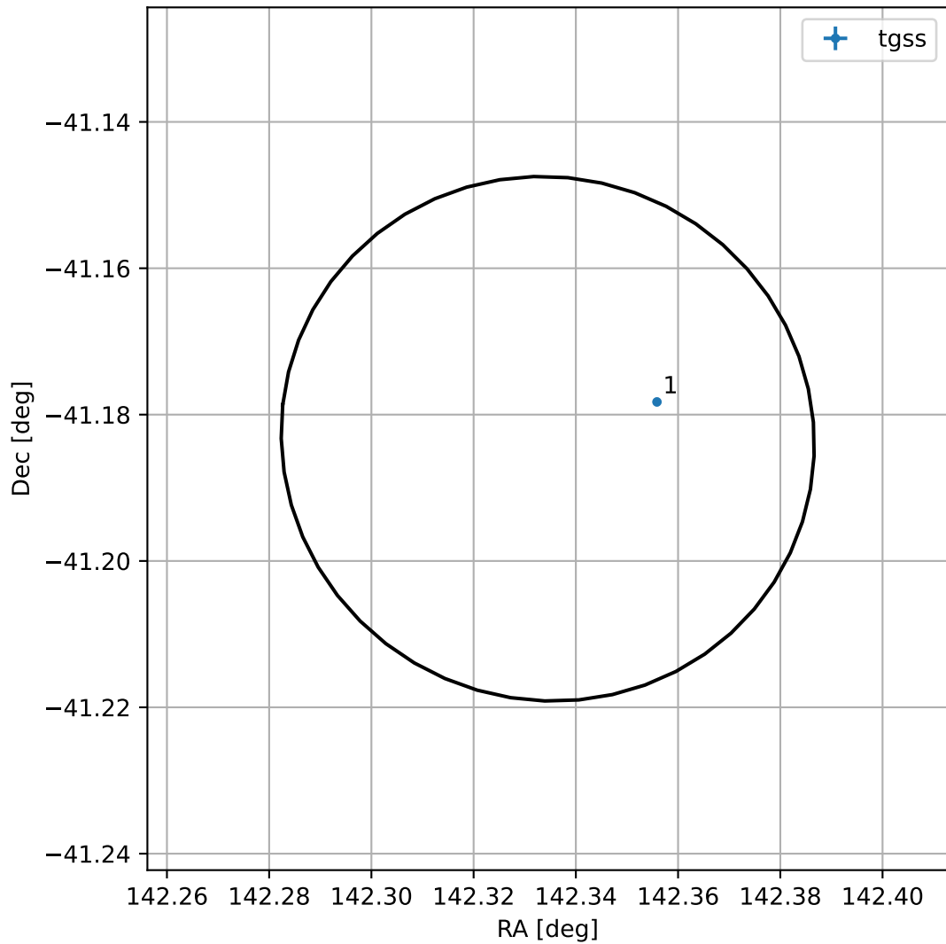
4FGL J0929.3-4110
