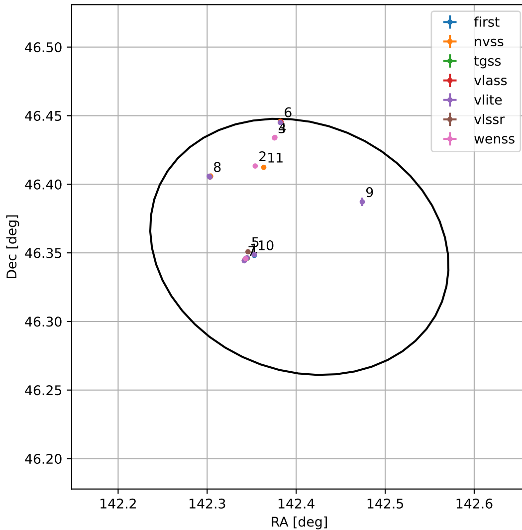
4FGL J0929.6+4621
