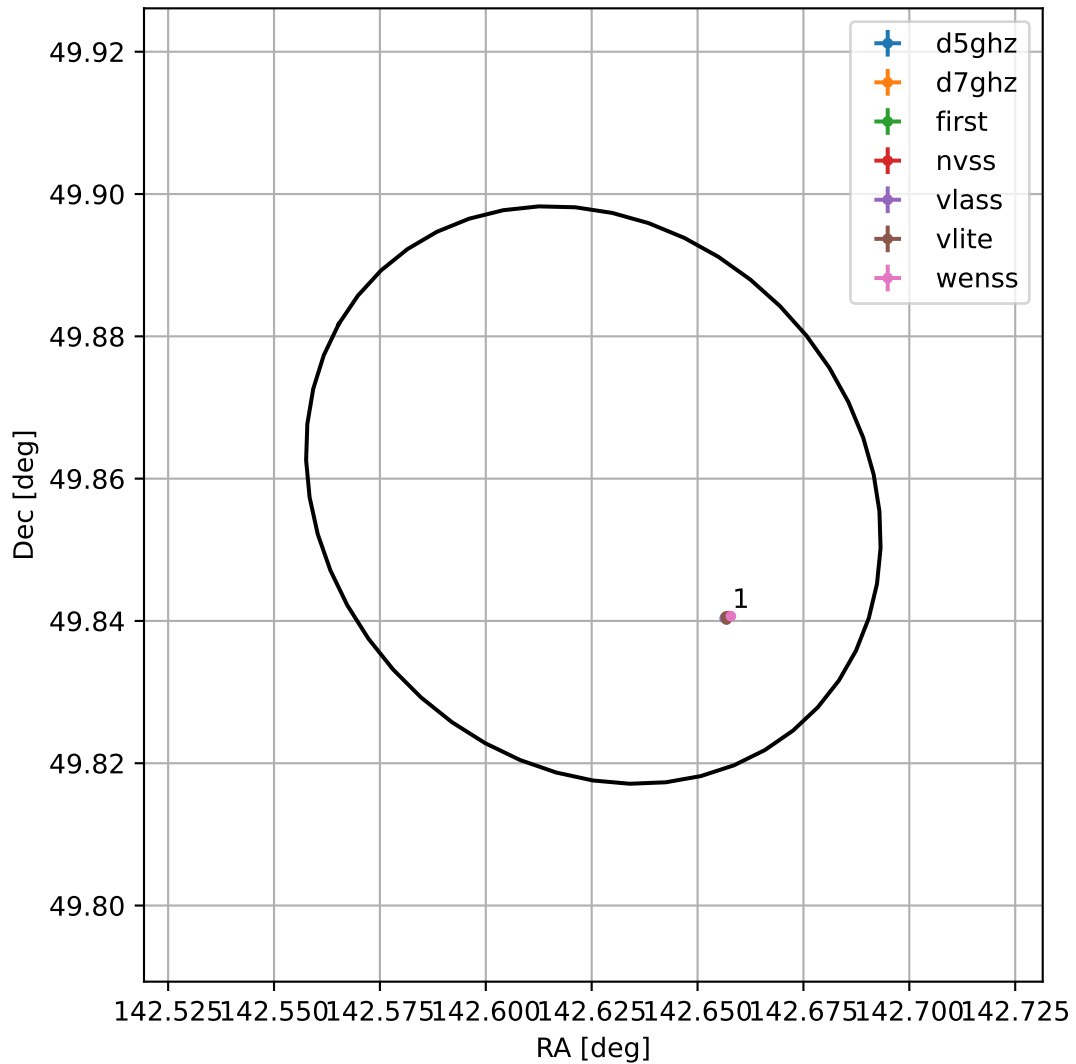
4FGL J0930.5+4951
