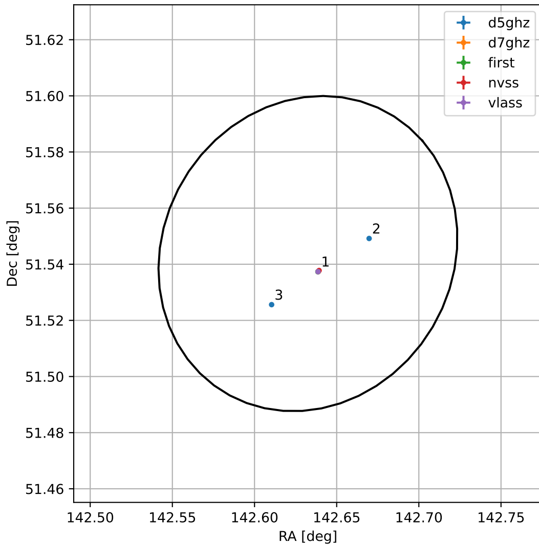
4FGL J0930.5+5132
