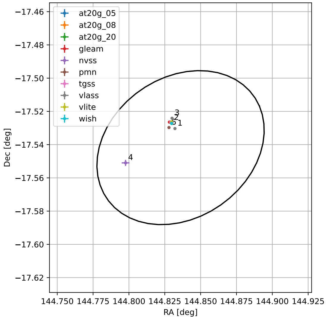
4FGL J0939.3-1732
