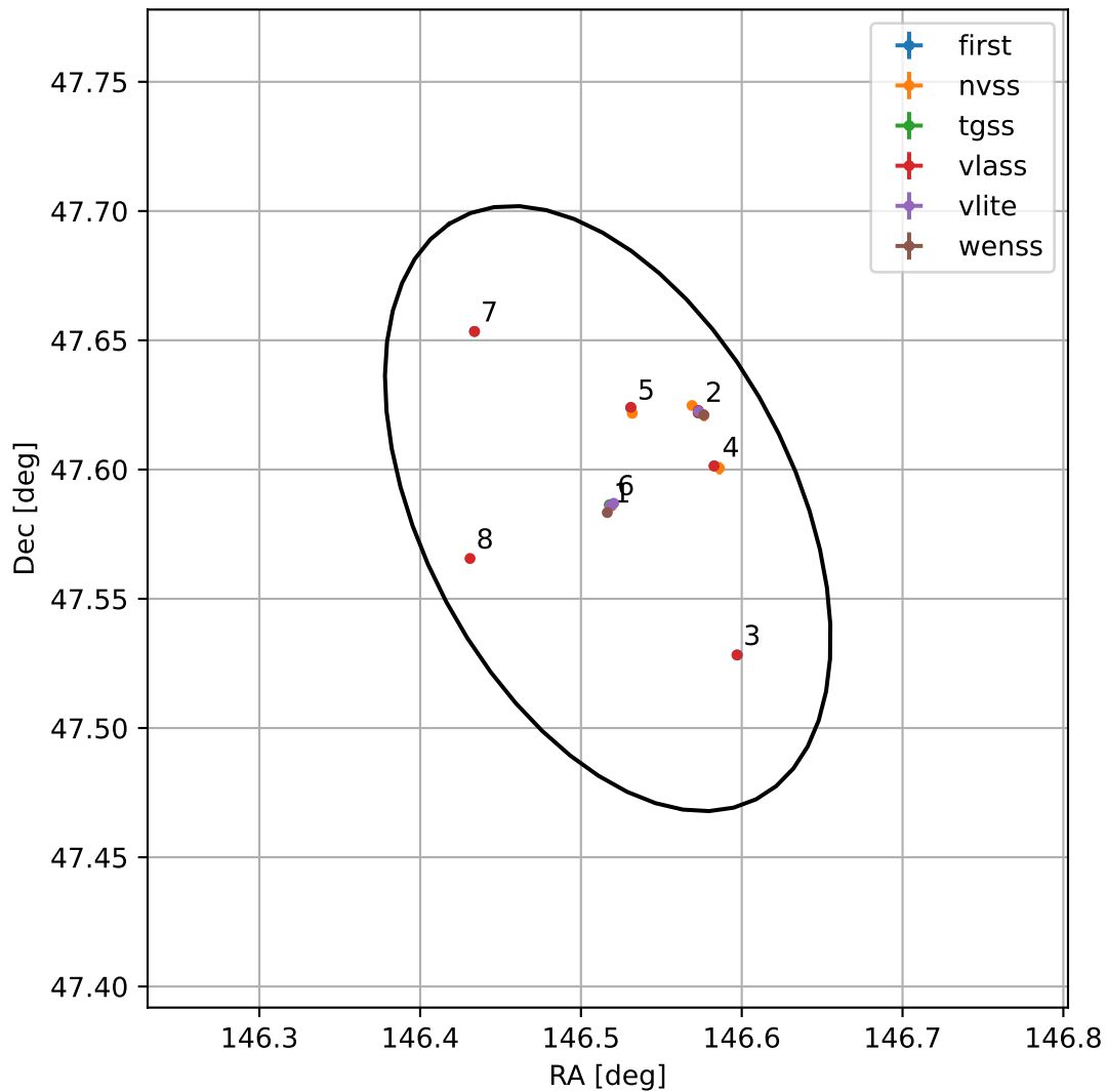
4FGL J0946.0+4735
