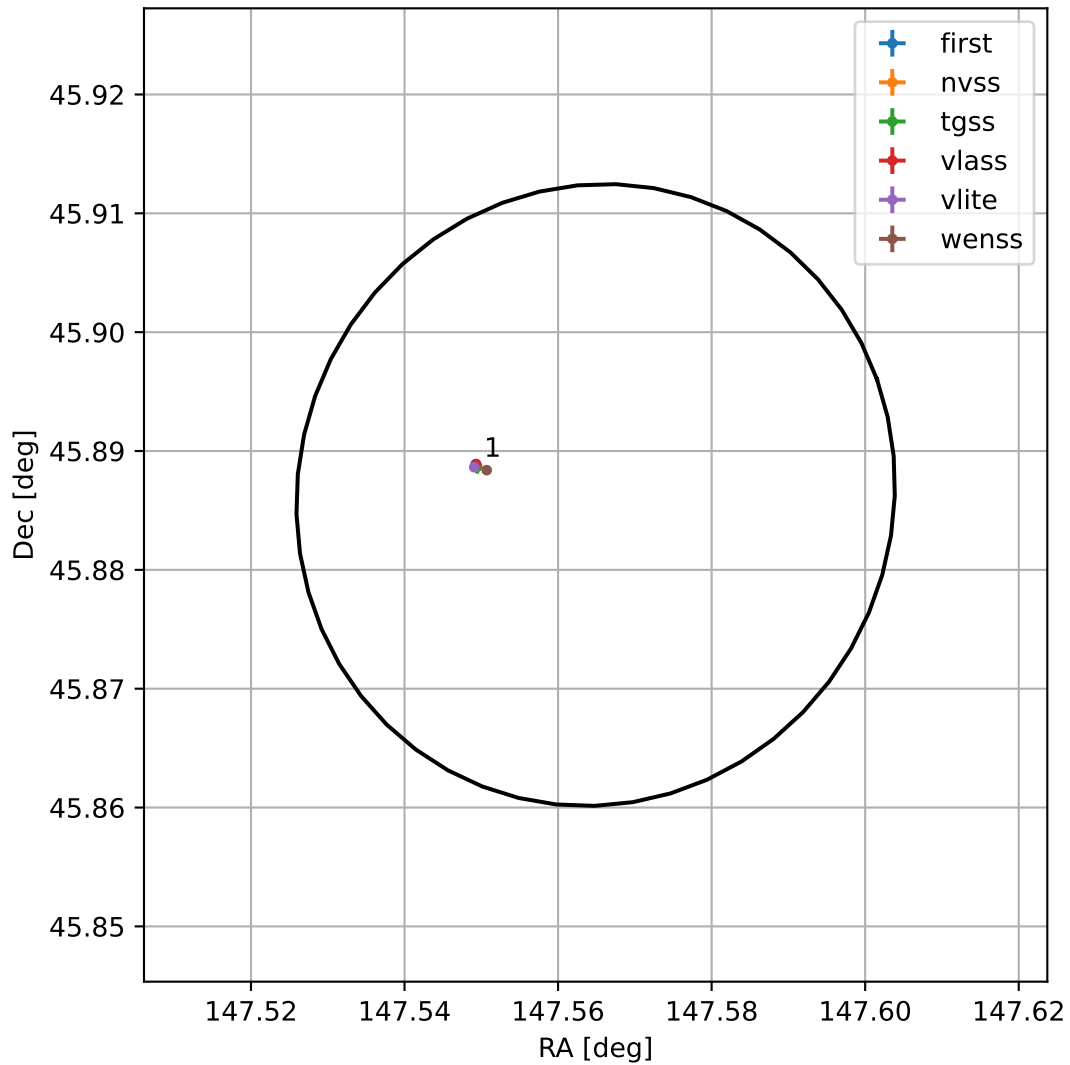
4FGL J0950.2+4553
