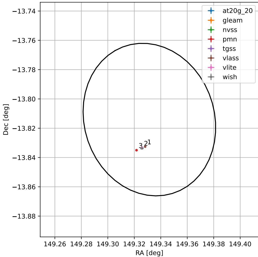
4FGL J0957.3-1348
