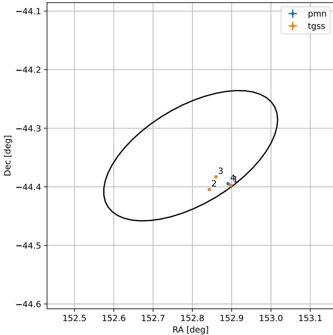
4FGL J1011.1-4420
