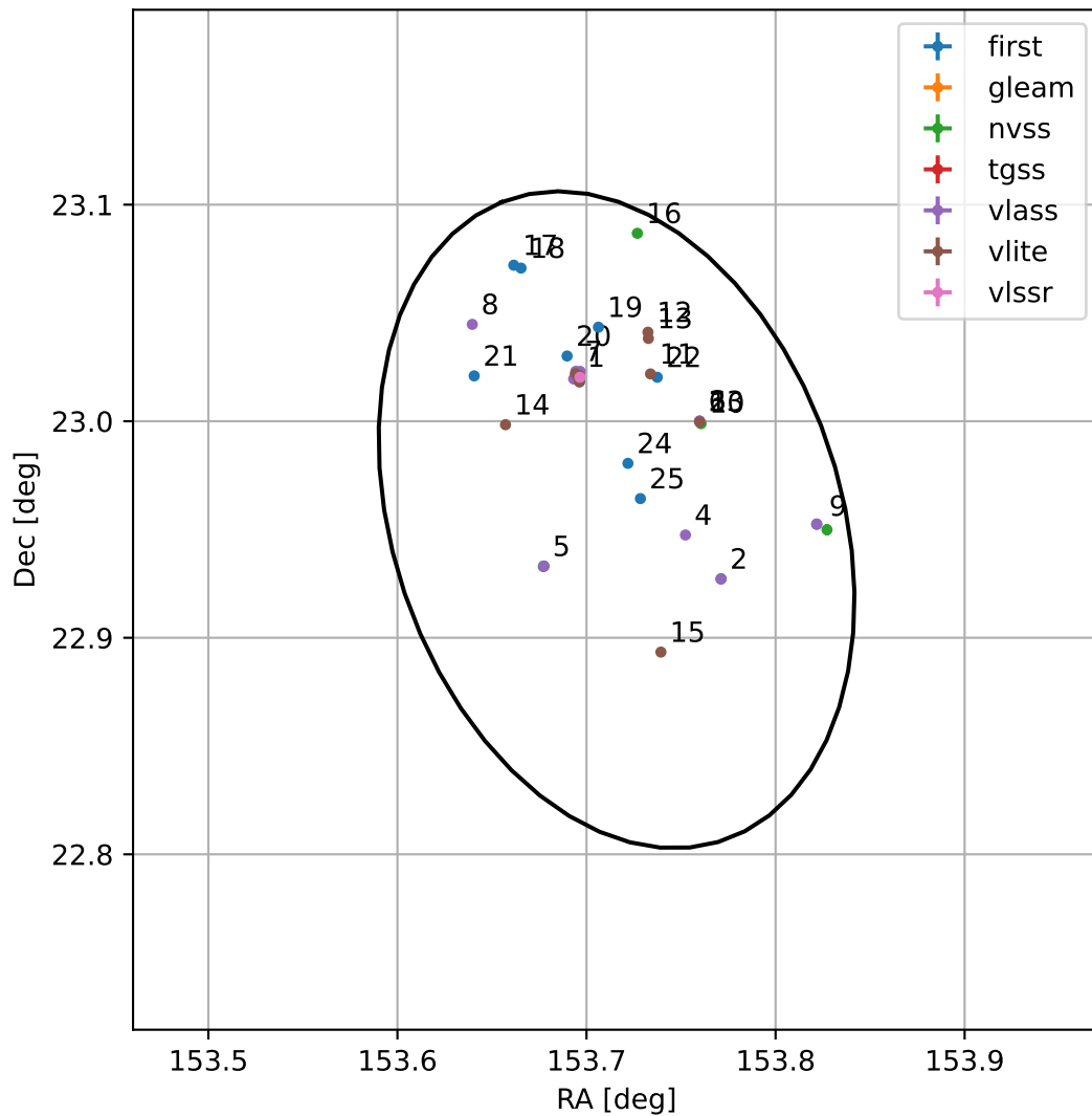
4FGL J1014.8+2257
