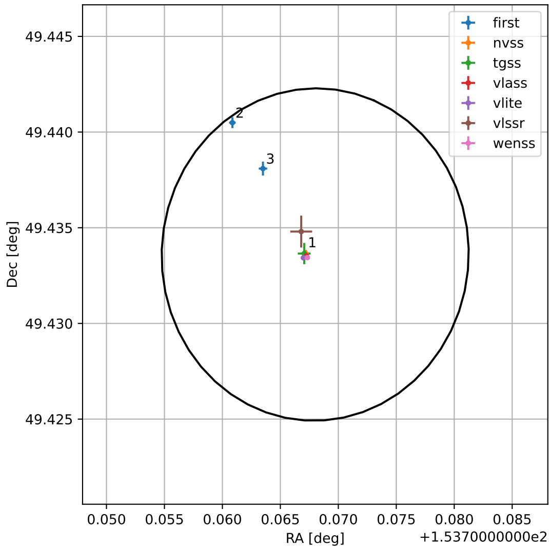
4FGL J1015.0+4926
