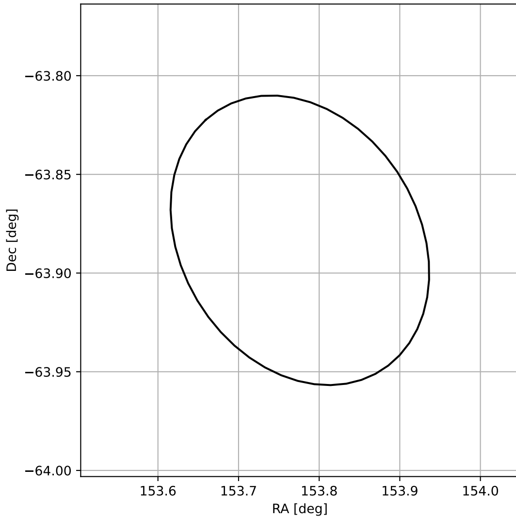
4FGL J1015.1-6353
