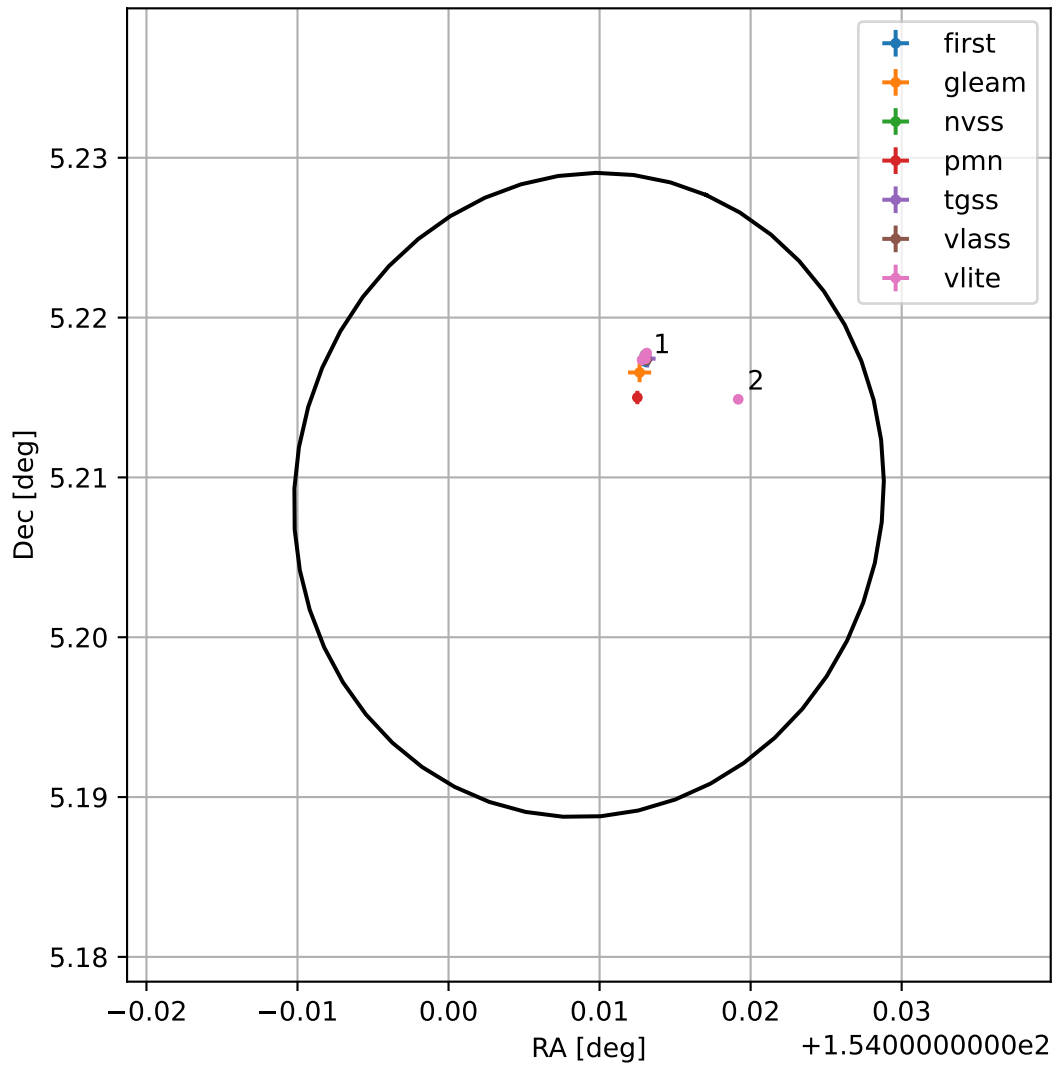
4FGL J1016.0+0512
