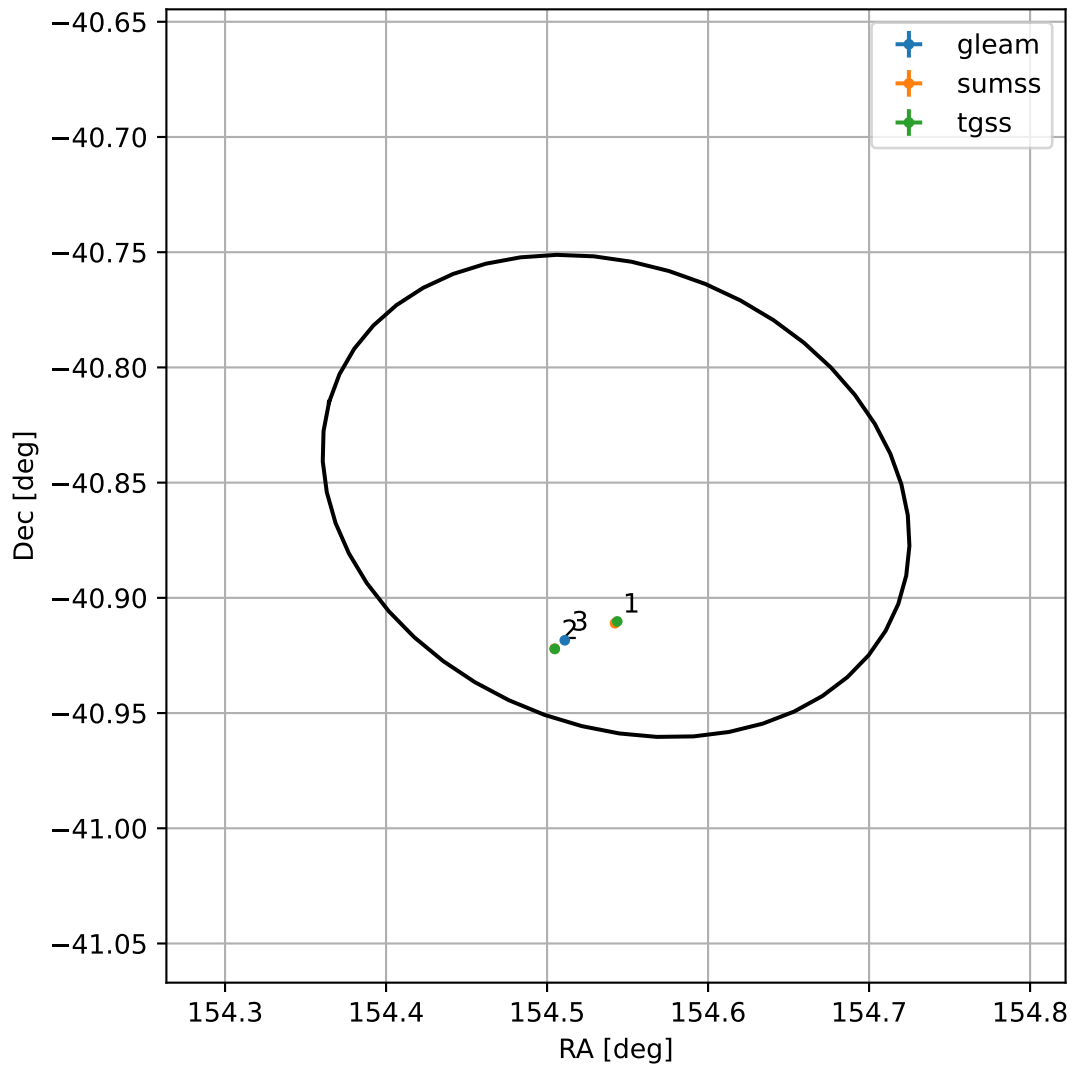
4FGL J1018.1-4051
