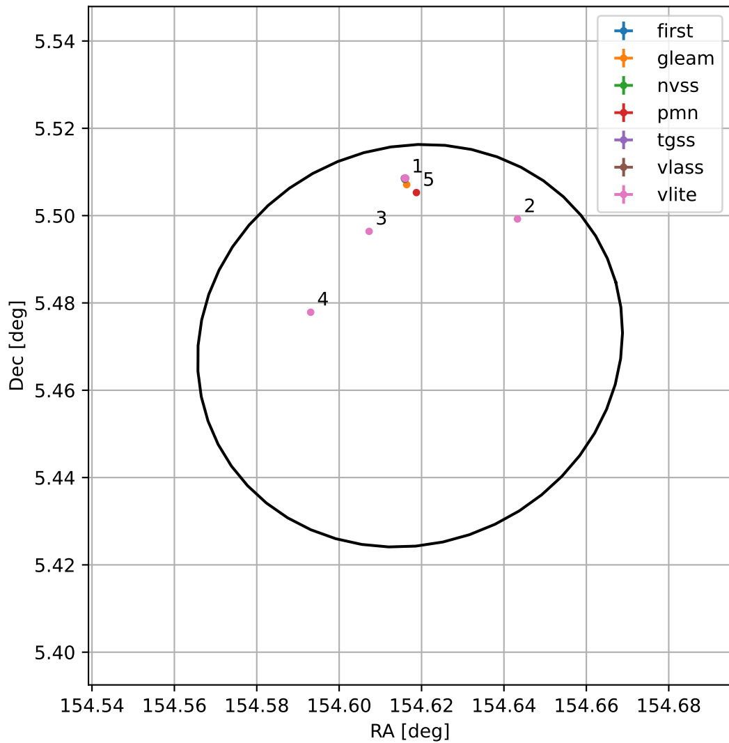
4FGL J1018.4+0528
