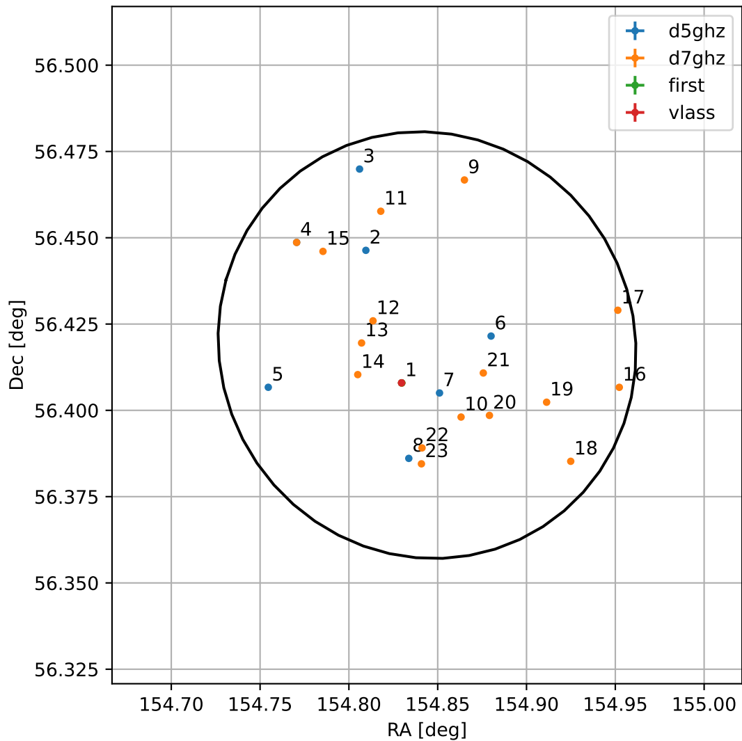
4FGL J1019.3+5625
