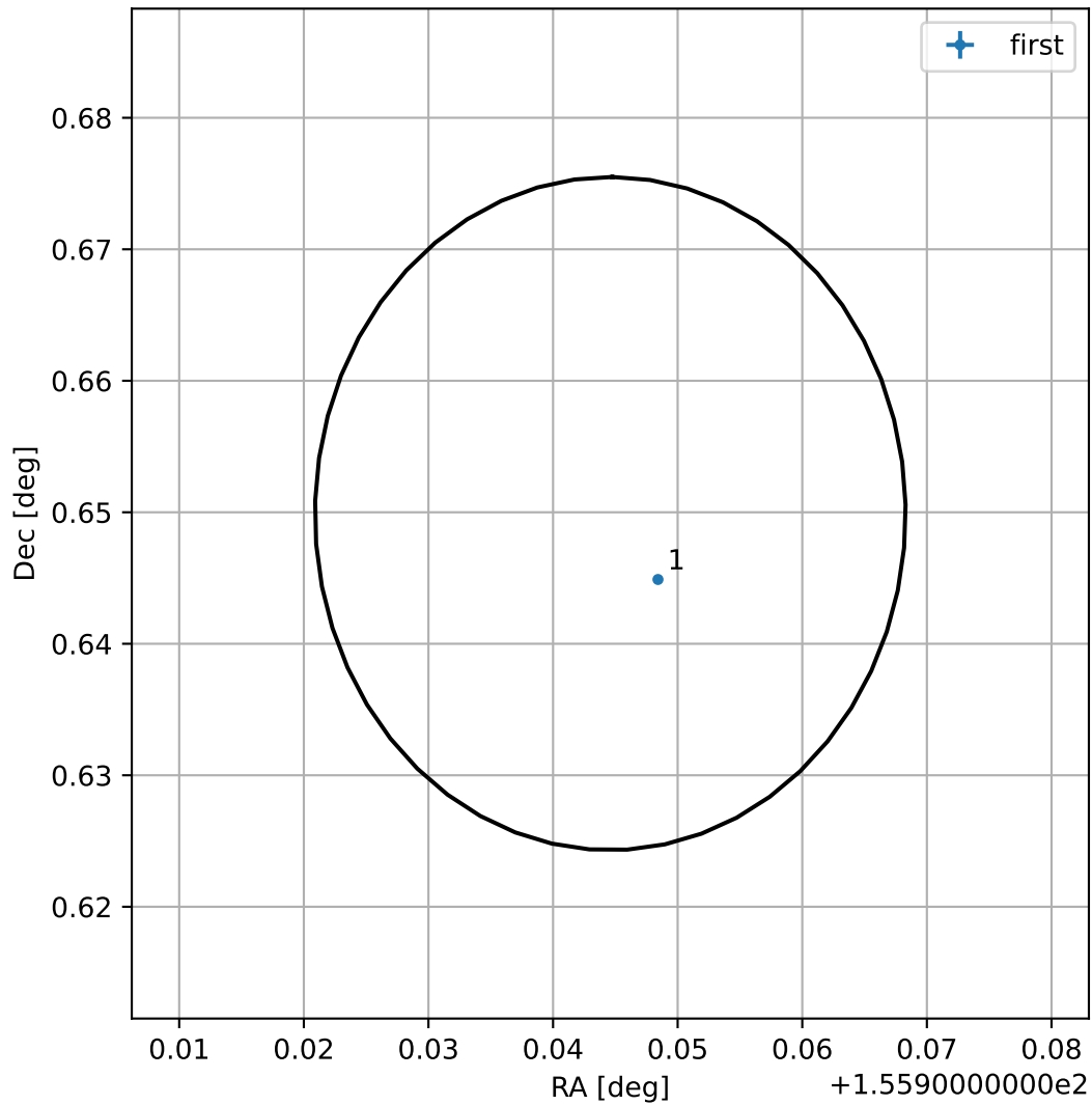
4FGL J1023.7+0038
