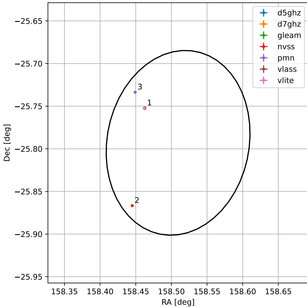
4FGL J1034.0-2547
