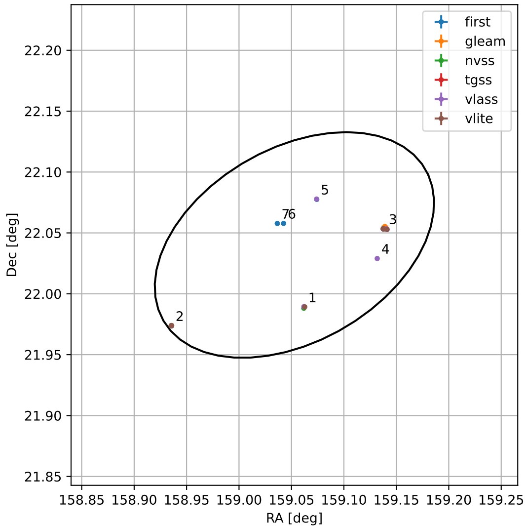
4FGL J1036.2+2202
