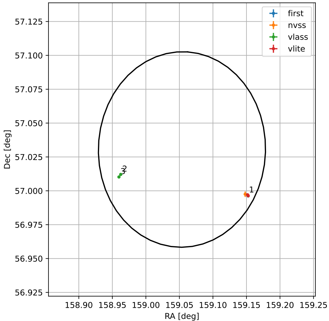
4FGL J1036.2+5701
