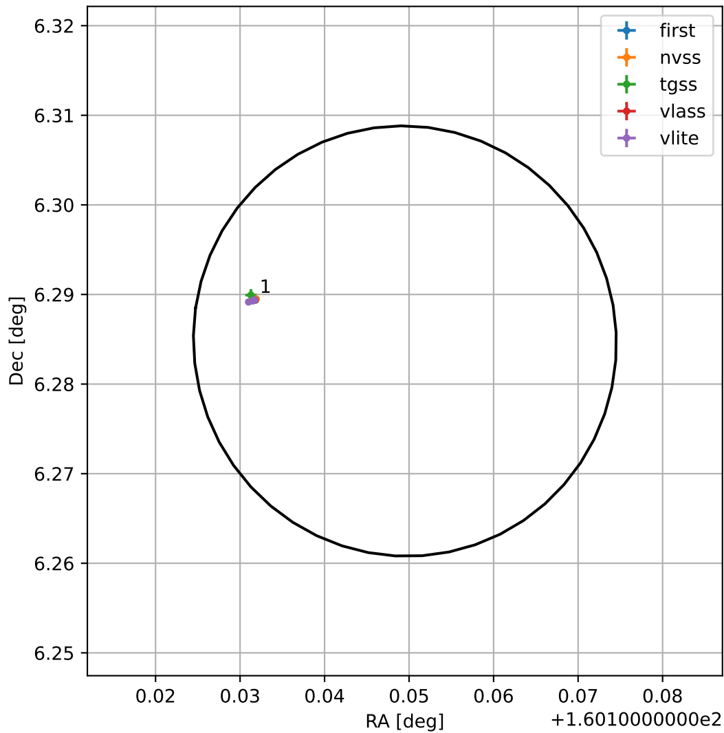
4FGL J1040.5+0617
