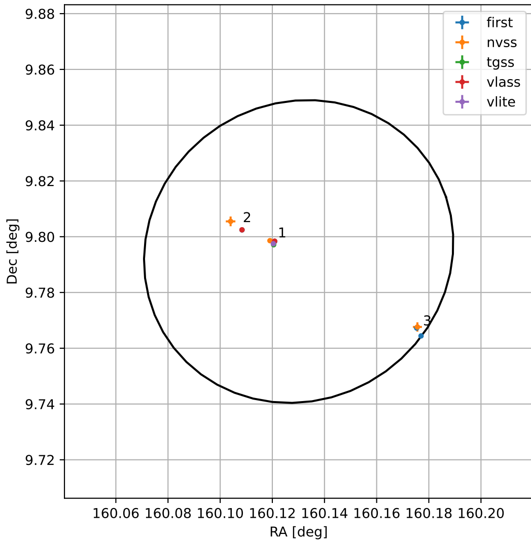
4FGL J1040.5+0947
