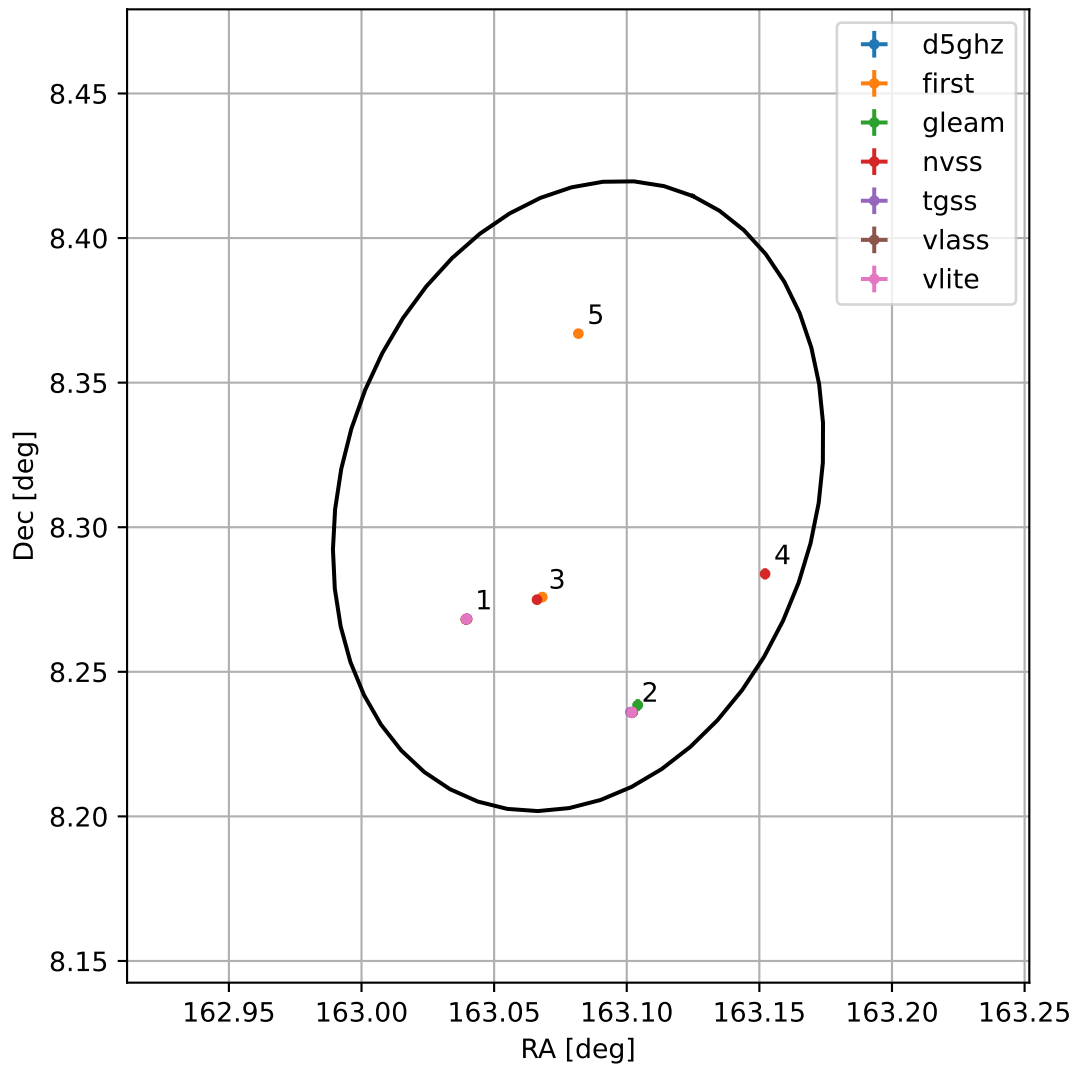
4FGL J1052.3+0818
