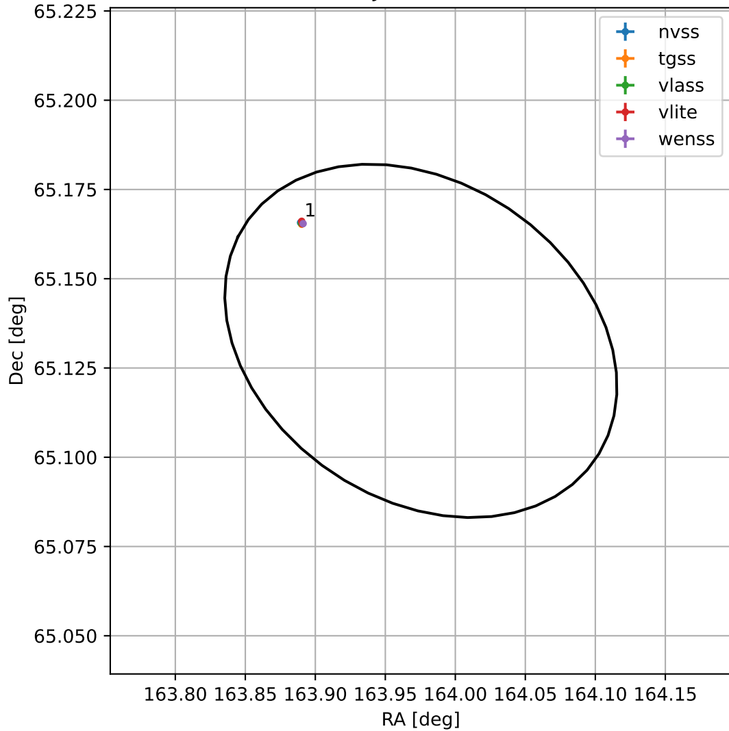
4FGL J1055.9+6507
