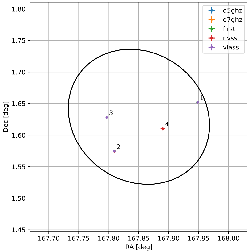
4FGL J1111.4+0137
