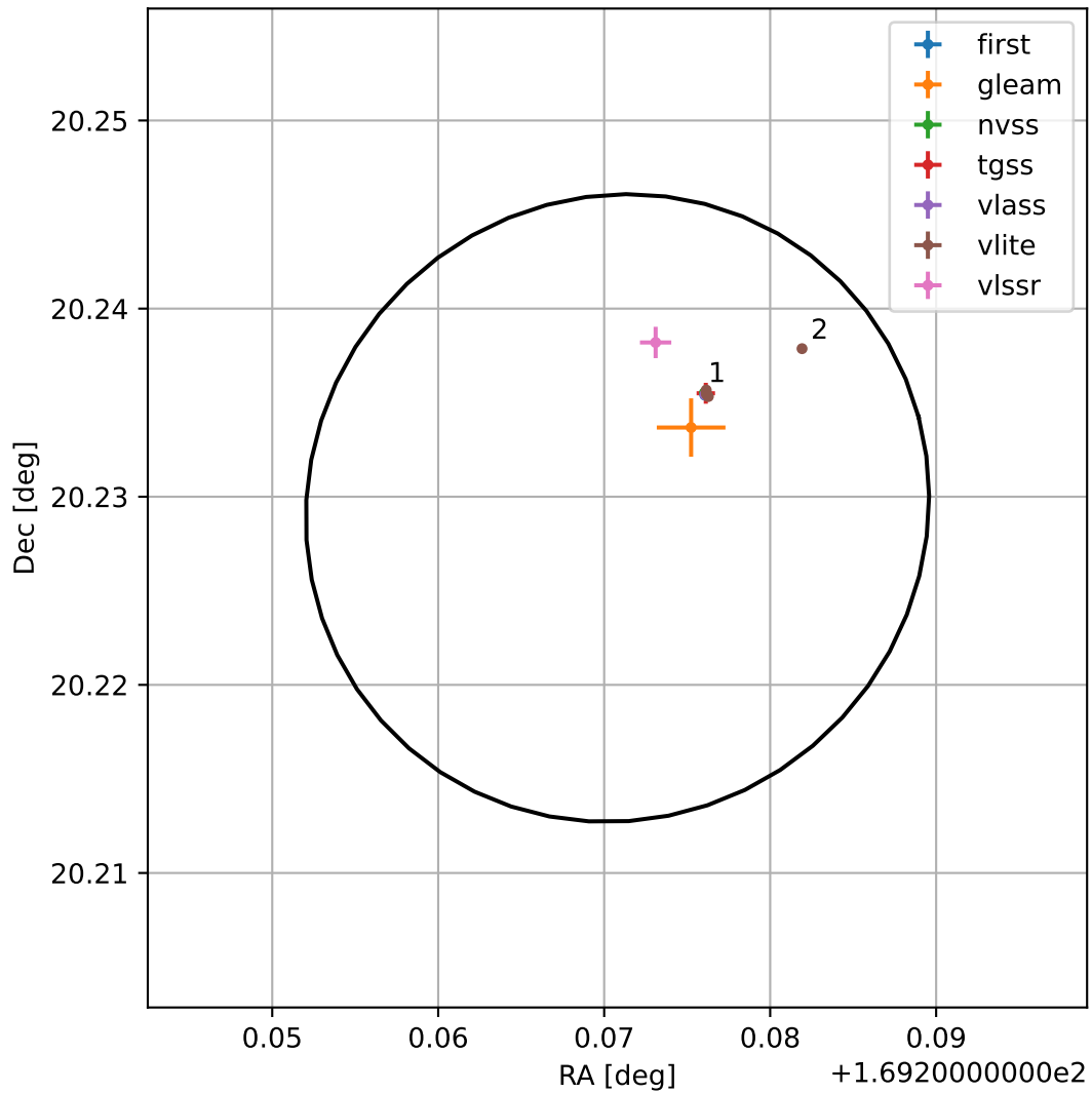
4FGL J1117.0+2013
