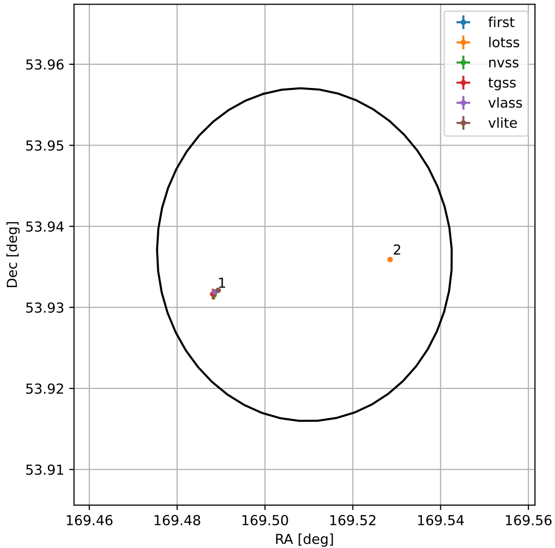
4FGL J1118.0+5356
