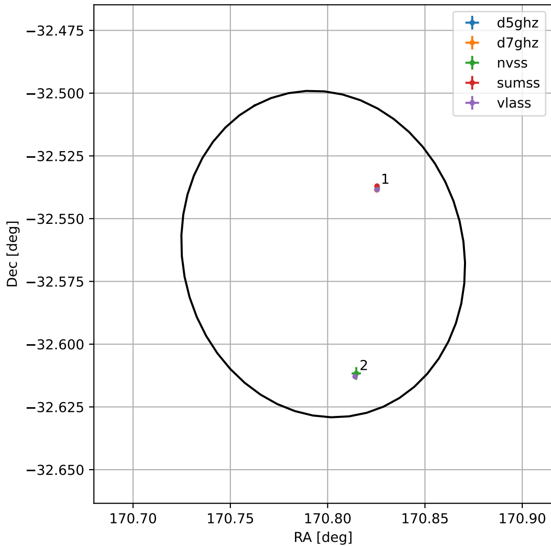
4FGL J1123.1-3233
