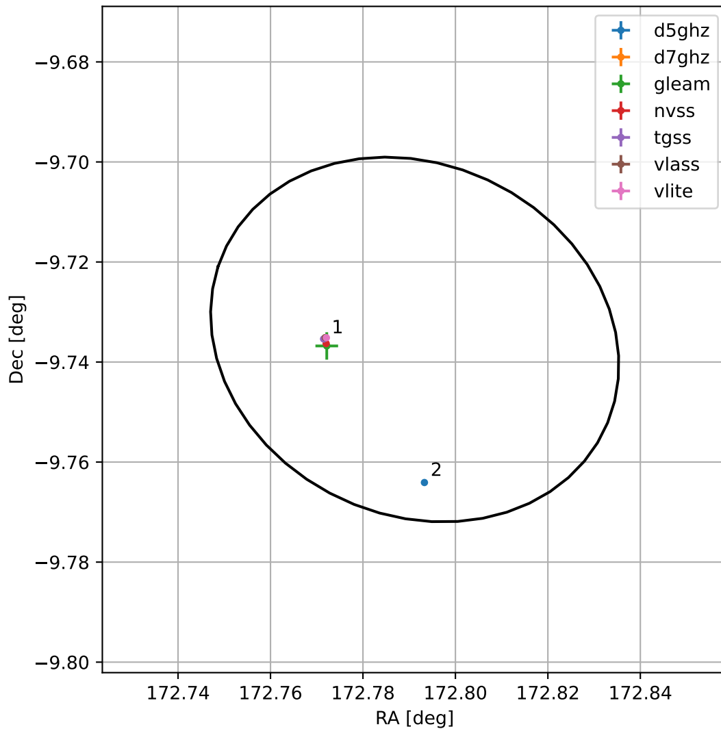
4FGL J1131.1-0944
